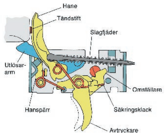
(3) Patronvis eld – Avfiring
