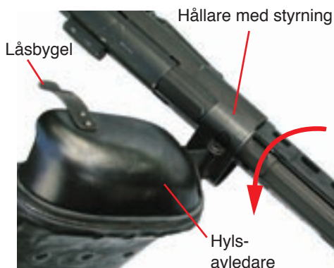
Fastsättning av hylsfångare Ak 4
