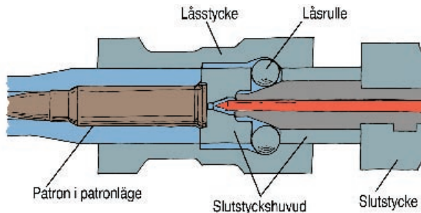
(1) Vapnet klart för eldgivning
