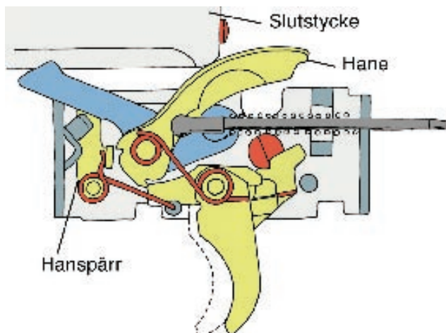
(5) Patronvis eld – Återgående rörelse
