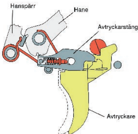
(2) Patronvis eld – Utgångsläge
